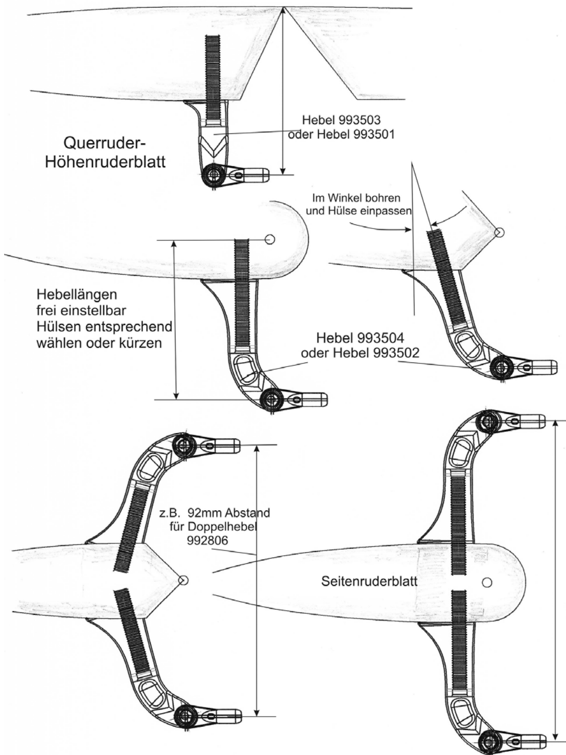
Einbaumöglichkeiten CFK Ruderhebel variabel
